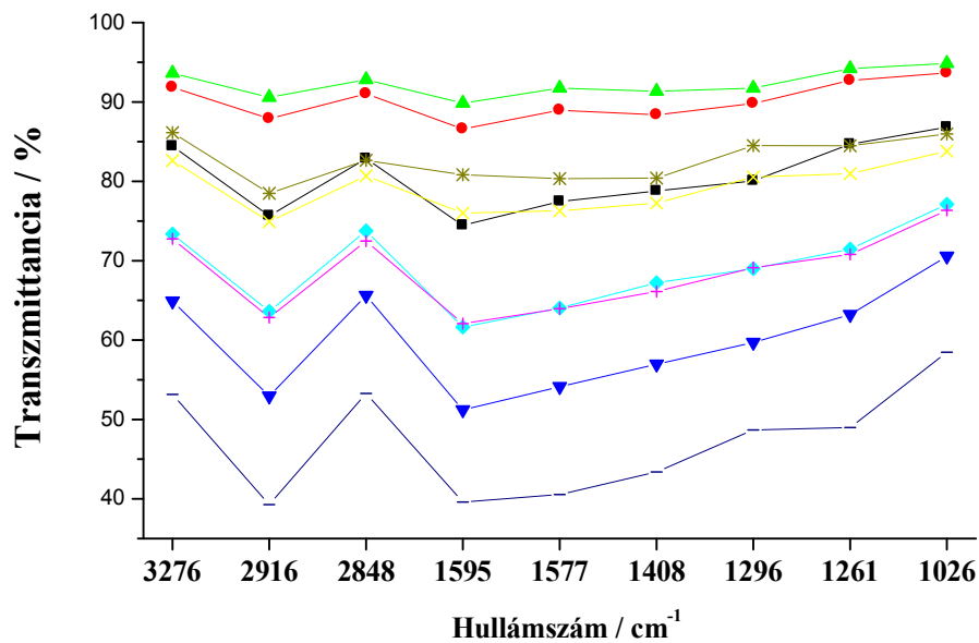
60. ábra A 4 hétig tárolt ostyák FTIR csúcsainak intenzitás-értékei (Színekódok: 1, 2, 3, 4, 5, 6, 7, 8, 9-es minta )
