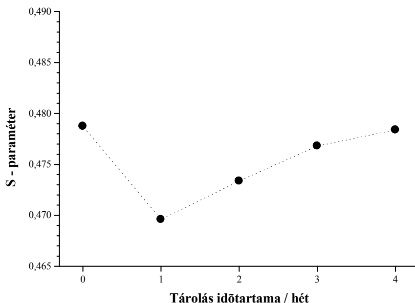
34. ábra A CP polimer S-paraméterének (DB mérés) változása a tárolás során
