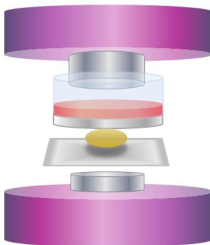
23. ábra A gél-film átmenet vizsgálatának PALS mérési elrendezése
