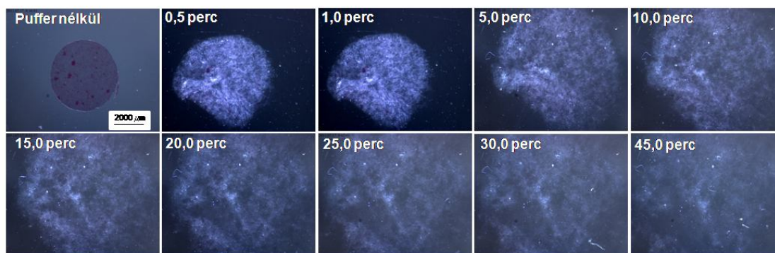
76. ábra Az öntött film viselkedése a kioldó közegben
