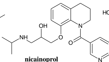
nicainoprol antiarrhythmic drug
